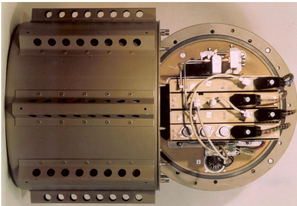
Az antennával egybeépíthető 8 GHz-es, KSR-8 típusjelű kiskapacitású analóg mikrohullámú adóvevő konténere és belső felépítése.
