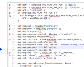
Megírom a kódot a LinkedIn API felhasználásával, a gépemre, vagy a felhőben
